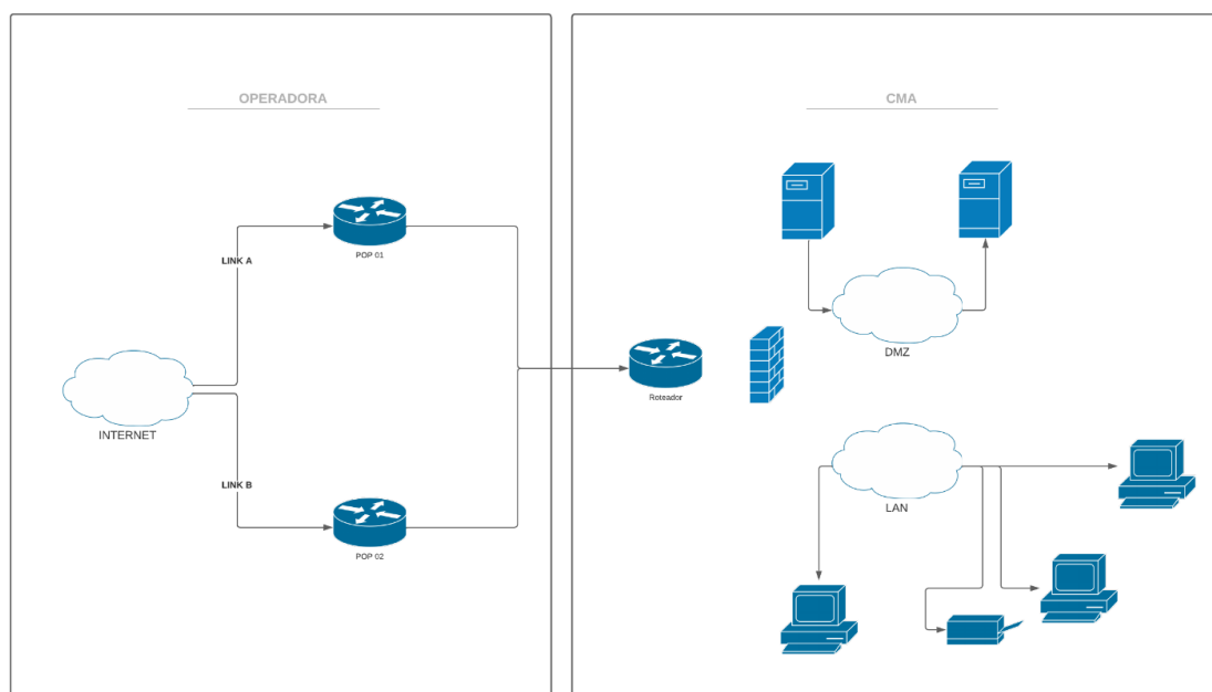
Figura 1 - Fibra ótica alta disponibilidade
